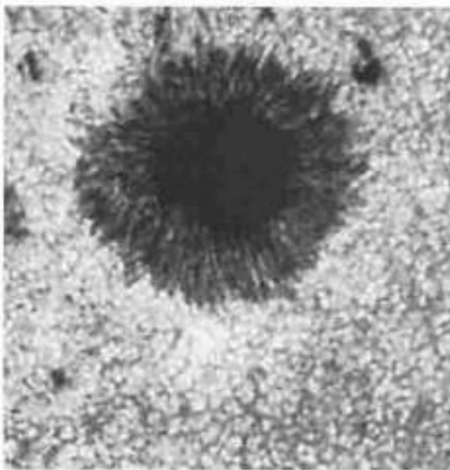
Figura 4. Mancha solar. Se observa la zona más oscura, umbra, rodeada de una zona más clara, penumbra. El estudio de la granulación existente en la fotosfera, determina la transmisión de energía de manera efectiva.
