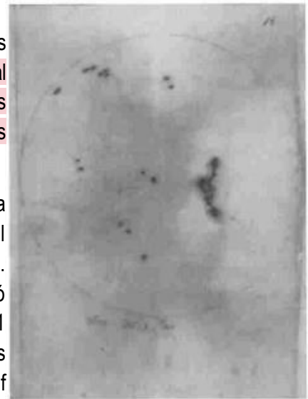
Figura 2. Dibujo de manchas solares realizado por Galileo Galilei en Sidereus Nuncius (mensajero de los astros).
